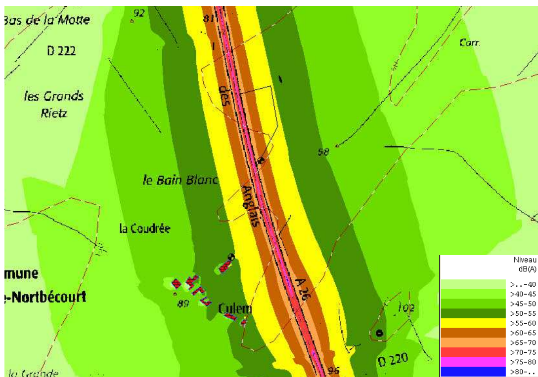
Figure 4 : Cartographie sonore hauteur = 2 m – Bruit Résiduel – Nuit
