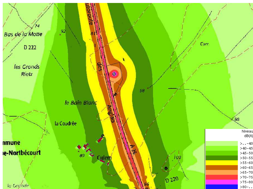
Figure 6 : Cartographie sonore hauteur = 2 m – Bruit Ambiant – Période Nuit
