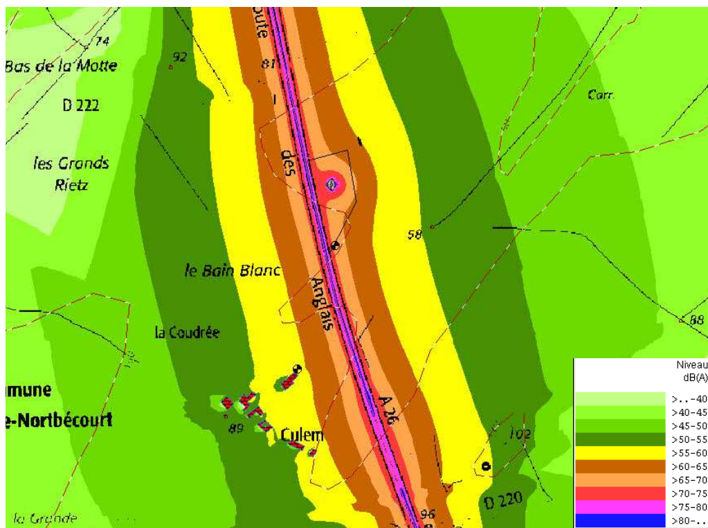
Figure 5 : Cartographie sonore hauteur = 2 m – Bruit Ambiant – Période Jour
