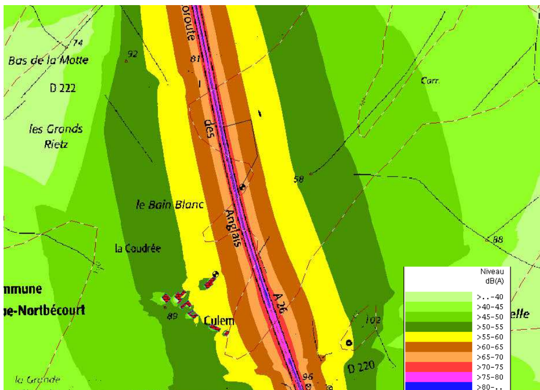
Figure 3 : Cartographie sonore hauteur = 2 m – Bruit Résiduel – Jour
